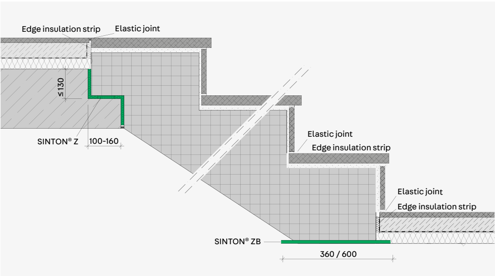
Systemschnitt Typ ZB
