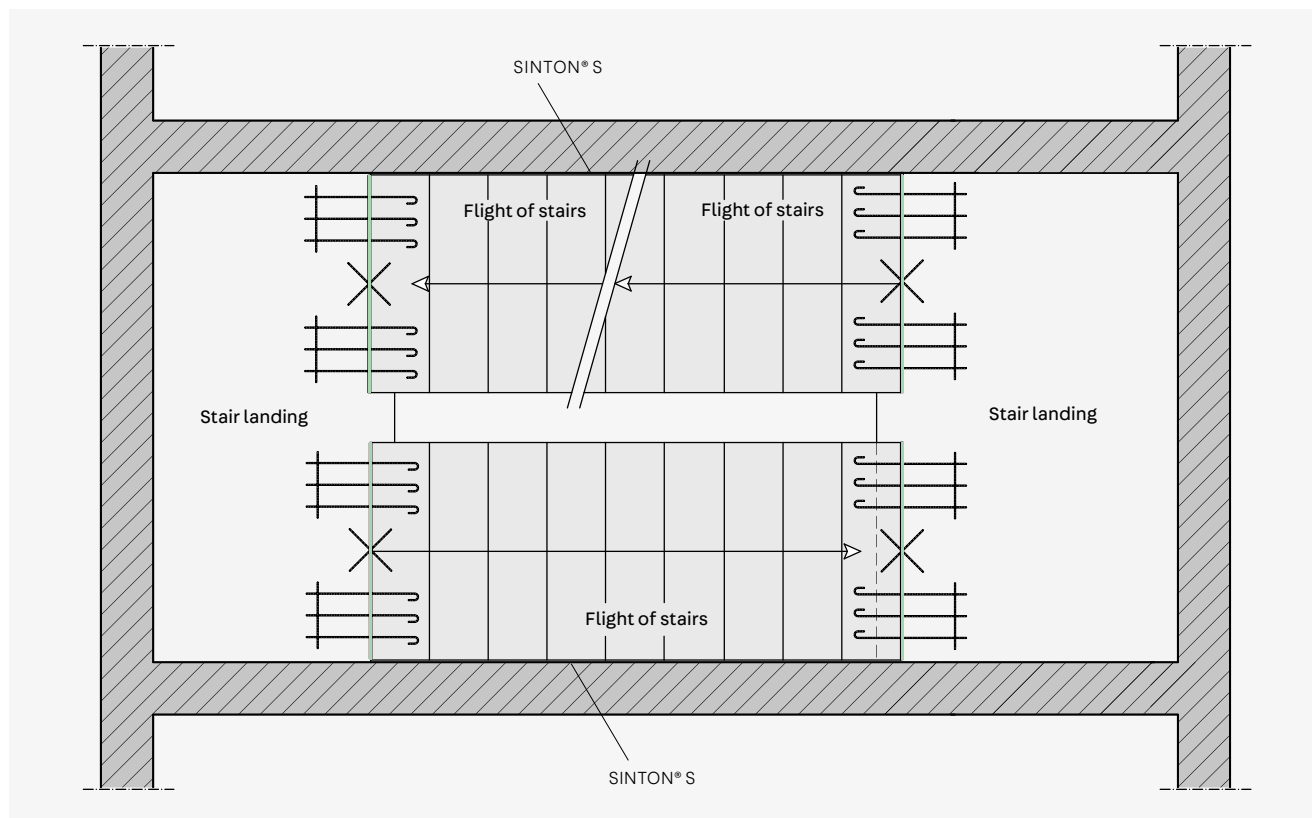
Anwendung des SINTON® HT-V im Podest in Kombination mit SINTON® S
